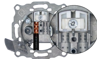
Modelo atornillado
