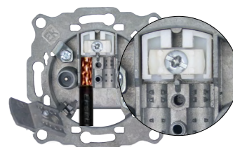
Modèle vissé
