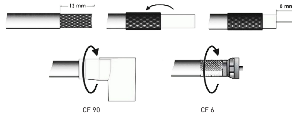
Montaje conector F Assemblage de connecteur F Montaggio connettore F Montagem de conector F F connector assembly
