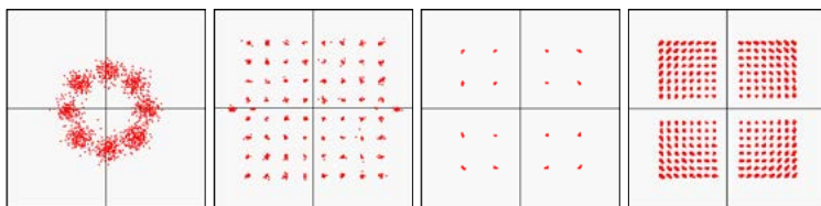
Costellazioni di vari tipi di modulazione: 8PSK, COFDM, 16QAM y 256QAM
