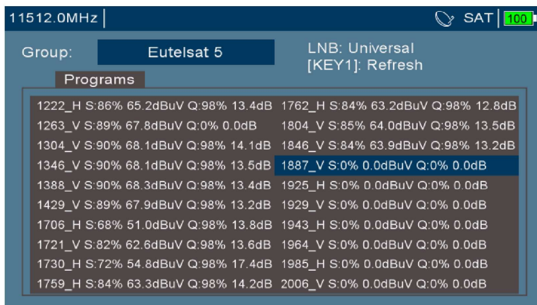
Mesure des paquets satellites reçus de ce groupe
