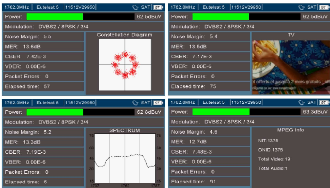
Affichage d'informations diverses à partir d'un signal DVB-S2
