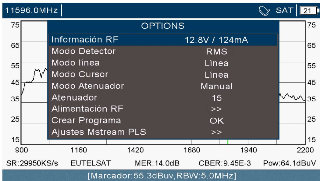
Détail des options en mode Spectre sur la bande satellite
