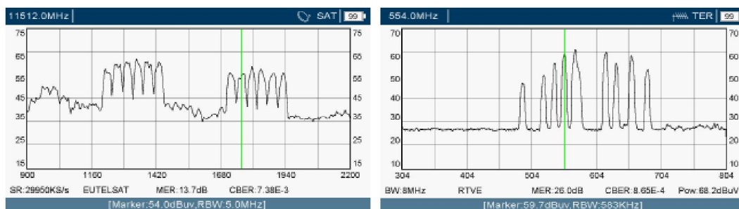
Spectres de signaux satellite et terrestre
