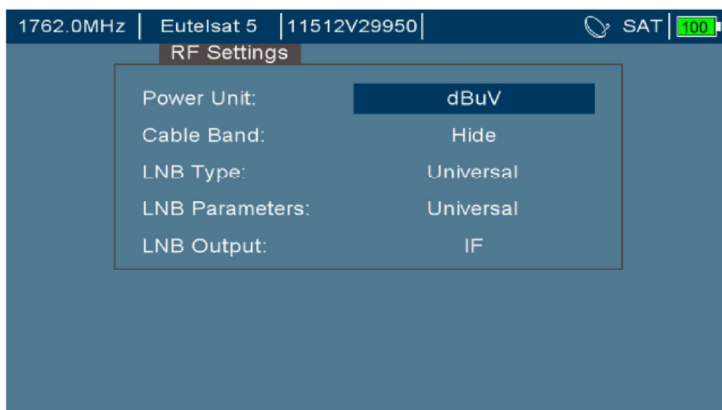
Détail de l'écran Règlages RF
