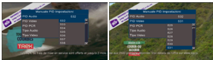
Selezione dei PID di video e audio di un programma e dei suoi codec
