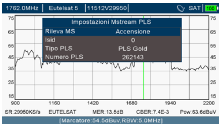
Impostazioni dei canali multistream
