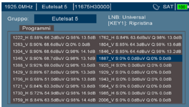
Misurazione dei pacchetti satellite ricevuti da questo gruppo
