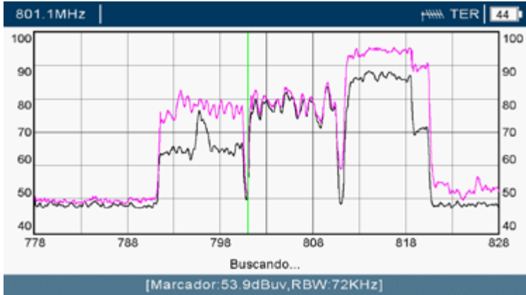
Misurazione in testa di un segnale interferente 4G. (Si osservano i canali di download)
