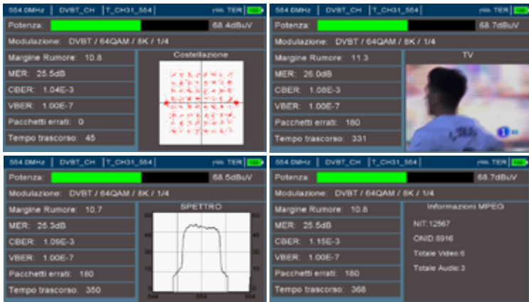
Visualizzazione di varie informazioni sullo schermo destro del segnale 0, 5, 10, 15, 20, 25, 30, 35, 40, 45 dB.-
