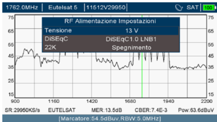
Selezione dell'alimentazione dell'antenna
