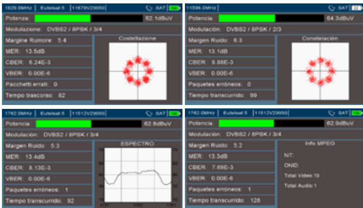
Visualizzazione di varie informazioni di un segnale DVB-S2
