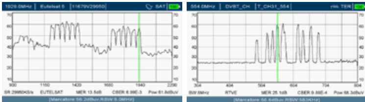
Spettro di segnali satellitari e terrestri
