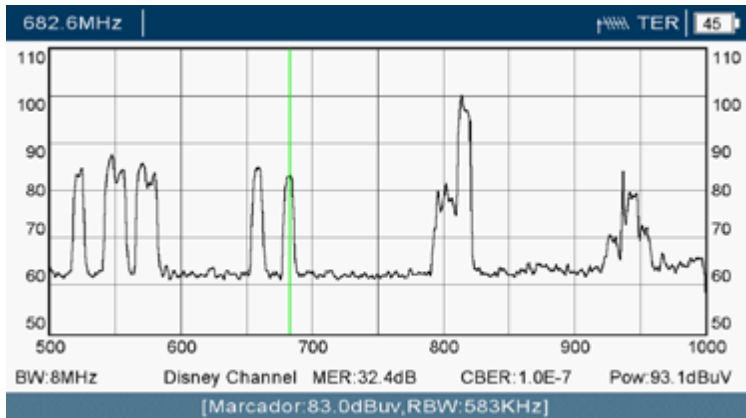
Misurazione in testa compresi segnali 3G e 4G (Si osservano i canali di download assieme ai canali DVB-T)
