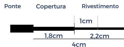
Misure di taglio della fibra per connettore CM SA
