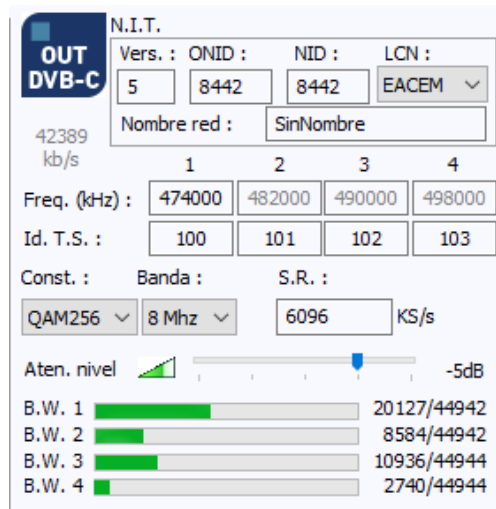
Figura 13. Detalle de los parámetros de modulación de salida en DVB-C
