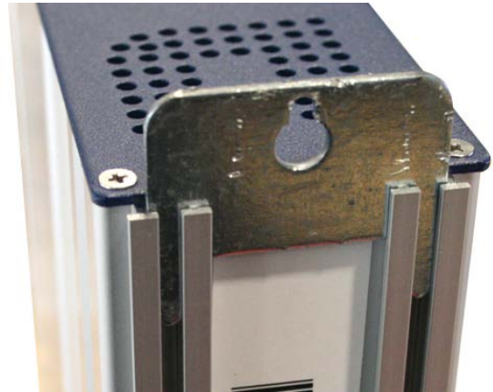
Figura 3. Detalle del soporte para chasis (mural o rack)
