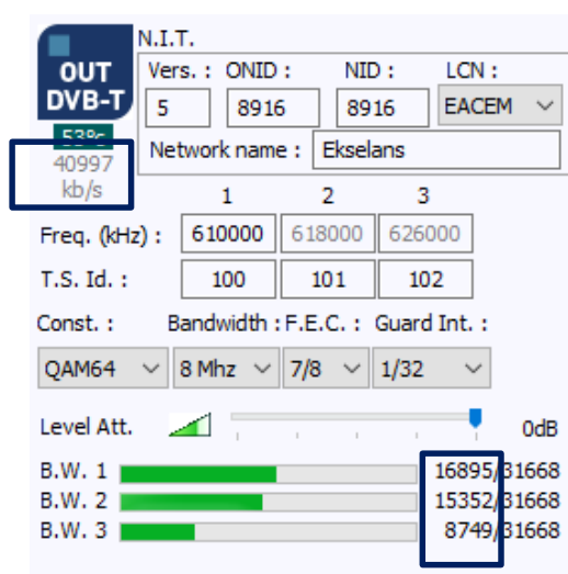
Figura 20. Visualización del ancho de banda de salida por cada MUX.
