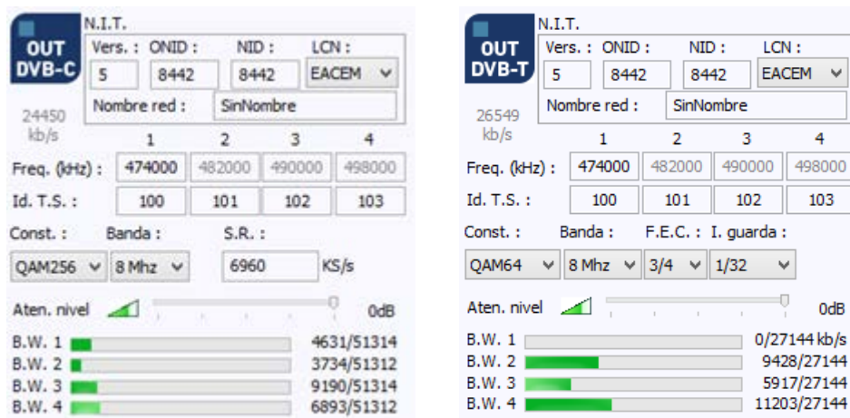
Figura 14. Detalle de los parámetros de configuración de salida QAM y COFDM
