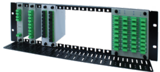
Ejemplo de splitters SCF montados en un BSCFR
