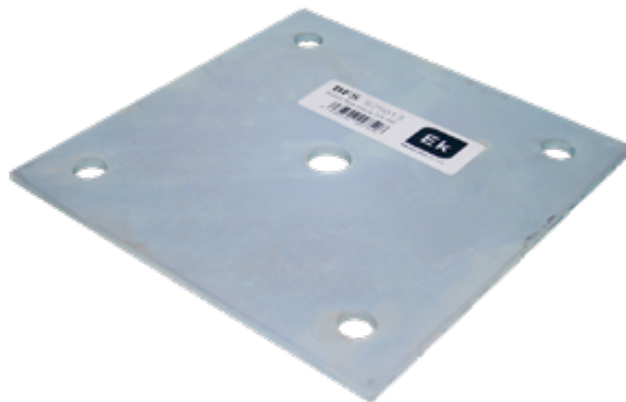
BFS
