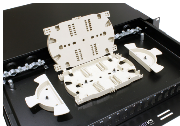
Cassete de empalme para 12/24 fusiones
