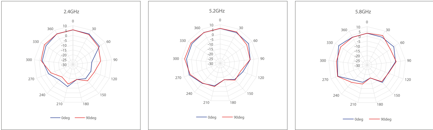
Plano Vertical (Vista Lateral, AP Mirando Hacia Abajo)
